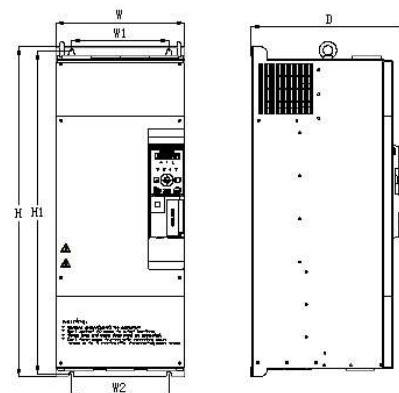
Рис. 3. IMD_E 18,5 – 30 кВт
