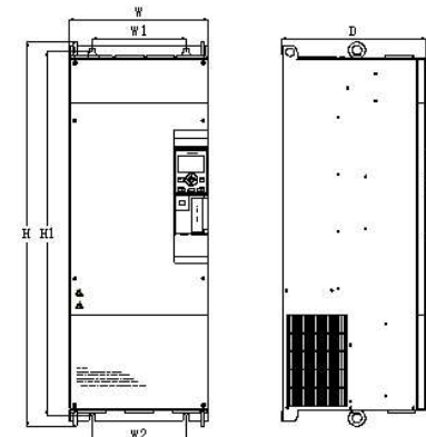
Рис. 4. IMD_E 37 – 200 кВт
